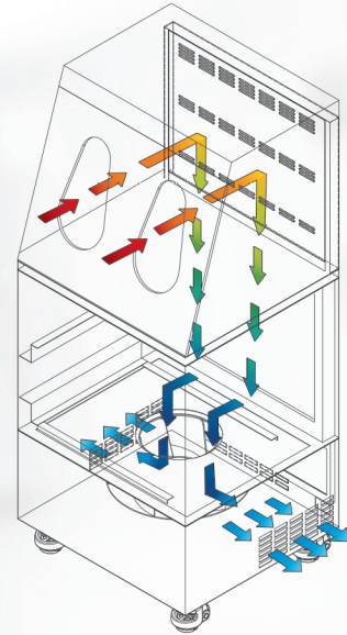
공기흐름도
